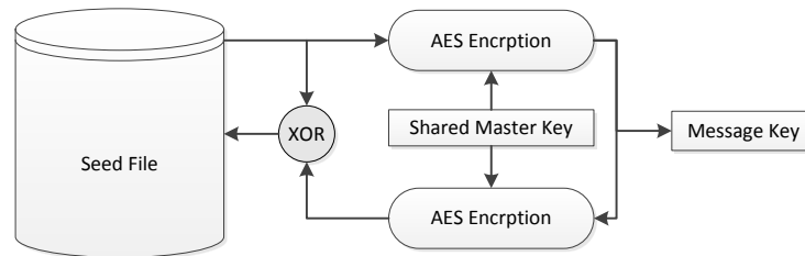
Fig. 5. Message Key Generation [23]
